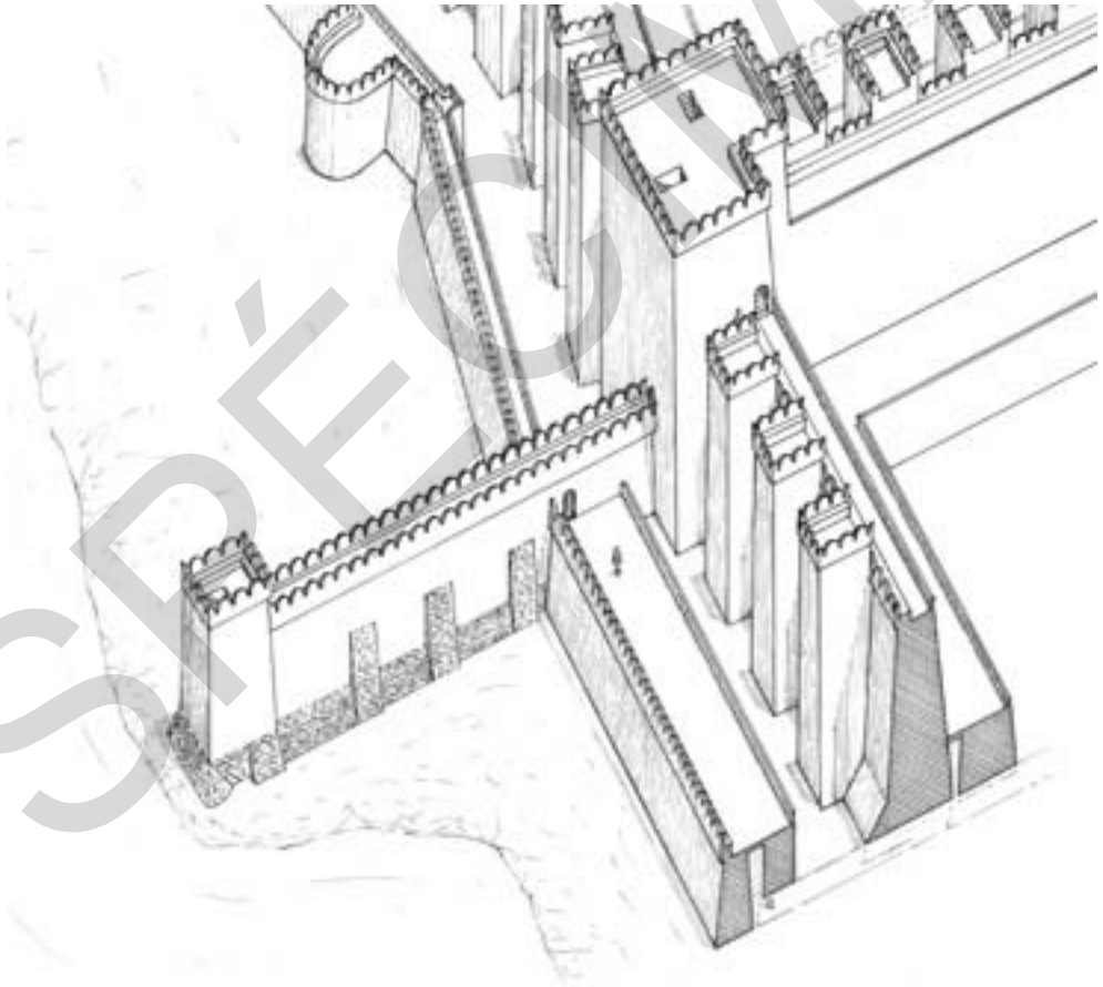
Fig. 78. Reconstitution du port de la forteresse d'Aniba (dessin de l'auteur)
